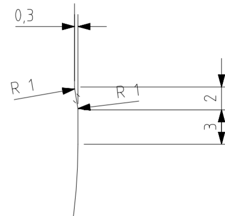
DETALLE D ESCALA 3:1
