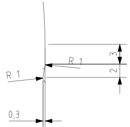
DETALLE C ESCALA 3:1
