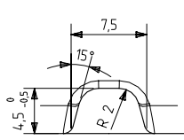
DETALLE T ESCALA 3:1
