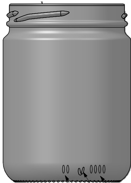
VISTA FRONTAL (FRONT VIEW) N° MODELO (JOB No) ANAGRAMA (PUNTMARK VIDRALA) N° MOLDE (CAVITY NUMBER)
