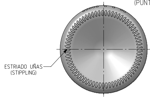
VISTA DEL FONDO (BOTTOM VIEW)
