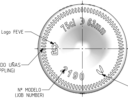
VISTA DEL FONDO (BOTTOM VIEW)
