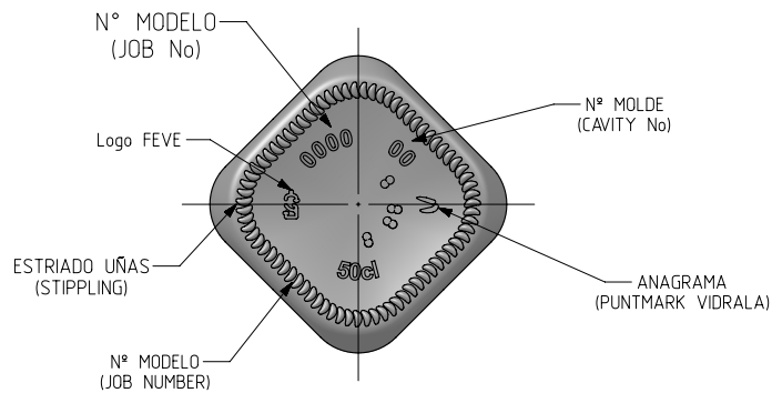
VISTA DEL FONDO (BOTTOM VIEW)
